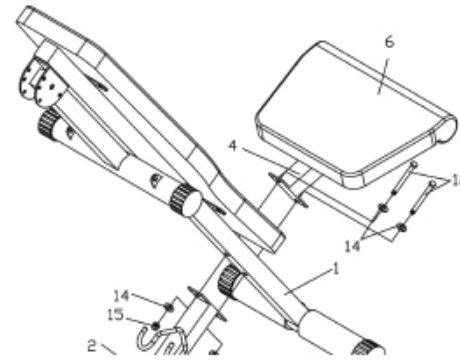
Rys. 2 Zamontuj wspornik z zamontowanym siedziskiem (#4) i tylną nogę (#2) na ramie głównej (#1) używając dwóch śrub (#12), czterech podkładek (#14) i dwóch nakrętek samozabezpieczających M10 (#15) tak jak to pokazano na rysunku.
